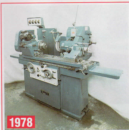
J. & S. 1300EIU UNIVERSAL GRINDER
